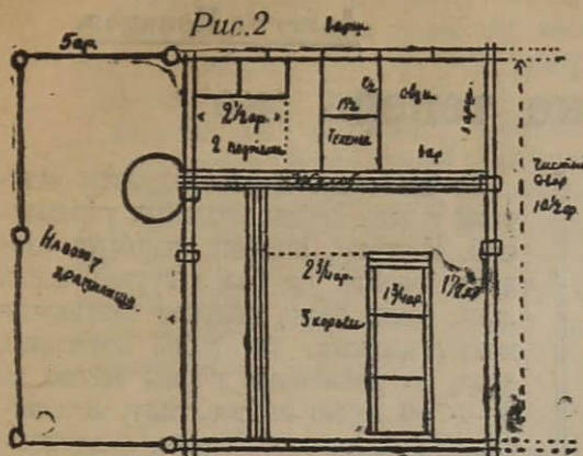
Рис. 2. План теплого двора при-над. Старина Григорьева С. Е., расчи-тан на 3 коров, 2 подтелков, 2 телят, и 2 — 3 овец или 1 поросенка. Раз-мер двора (внутри) 3,6 \times 6,7 мт. ( 8 \times 10\frac{1}{2} арш.). Позади двора распо-ложено навозохранилище размером 3,6 \times 6,7 мт. ( 5 \times 10\frac{1}{2} арш.), где по-мещается и сточный колодец для на-возной жижи. Навозохранилище пред-полагается с углублением на \frac{3}{4} арш. (0,5 мт.) в землю и над ним построй-ка крыши.
