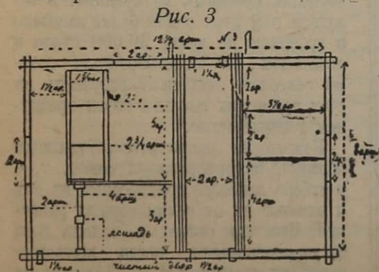
Рис. № 3. План теплого двора, пред-назначенного к постройке в дер. Би-рюково у гр-на Бобкова Д. А. Помеще-ние рассчитано на 3-х коров или 2-х коров и 1 подтелка, 1 лошадь, 2 по-росенка и 4 — 5 овец, размер двора 3,6 \times 8,9 мт. ( 8 \times 12\frac{3}{4} арш.). Навозо-хранилище и сточный колодец поме-щаются позади двора, углублено на 0,5 мт. ( \frac{3}{4} арш.) в землю без крыши. Все дворы отделяются от дома чи-стым двором. На первых двух помеща-ются лошади. Коровы и подтелки сто-ят на привязи без всяких перегородок и лишь на первое время допускается
